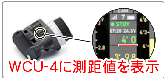
WCU-4のディスプレイに測距値が表示されます (写真はLDSレンズ使用時の表示です)
